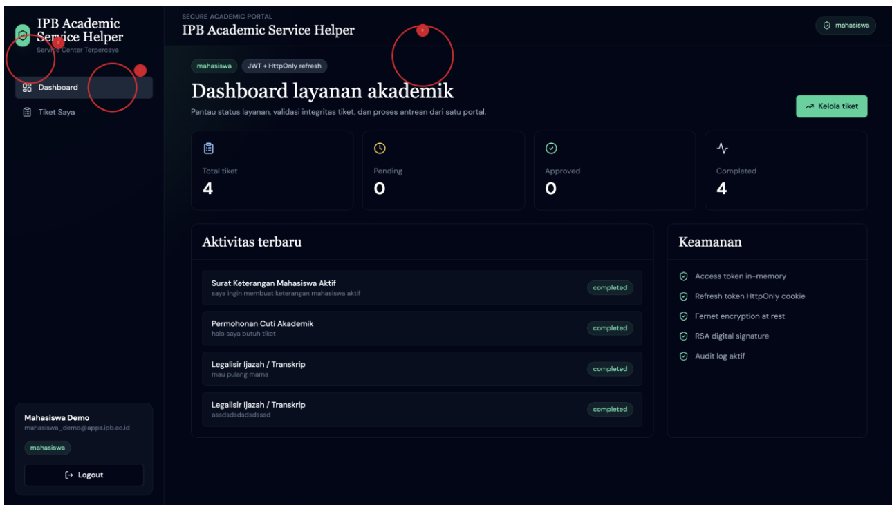
Gambar 2. Dashboard Mahasiswa
