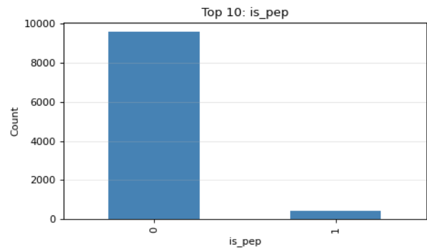
is_pep top 10
