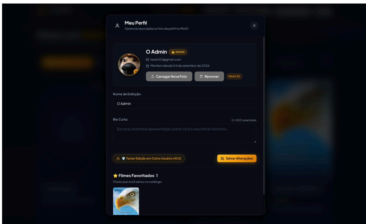
Figura 12: Atividade 6 — resultado funcional (perfil com foto no MinIO, bio, favoritos e verificação de segurança 403)
