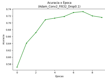
Adam – 32 filtros
