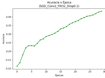
SGD – 32 filtros
