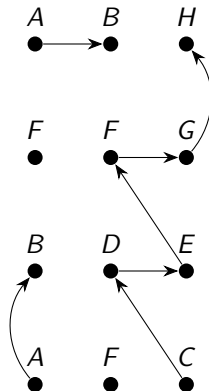
Figura: Grafo G.
