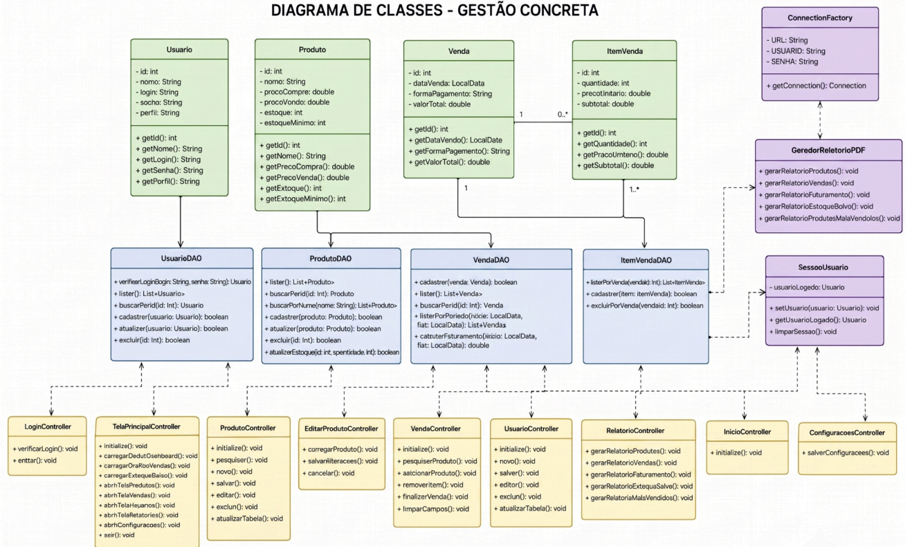
DIAGRAMA DE CLASSES - GESTÃO CONCRETA
