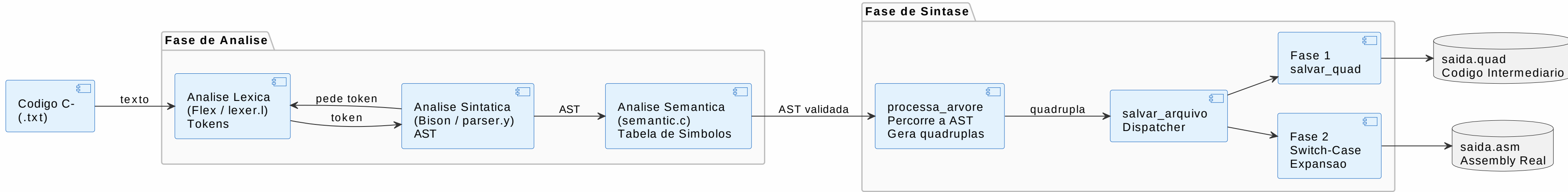
Diagrama de Blocos - Pipeline do Compilador C-
