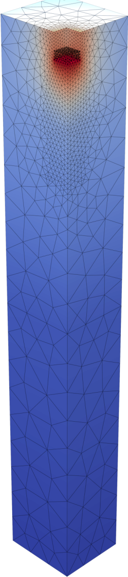
Asentamientos por Carga de Columna (Fase 2)
