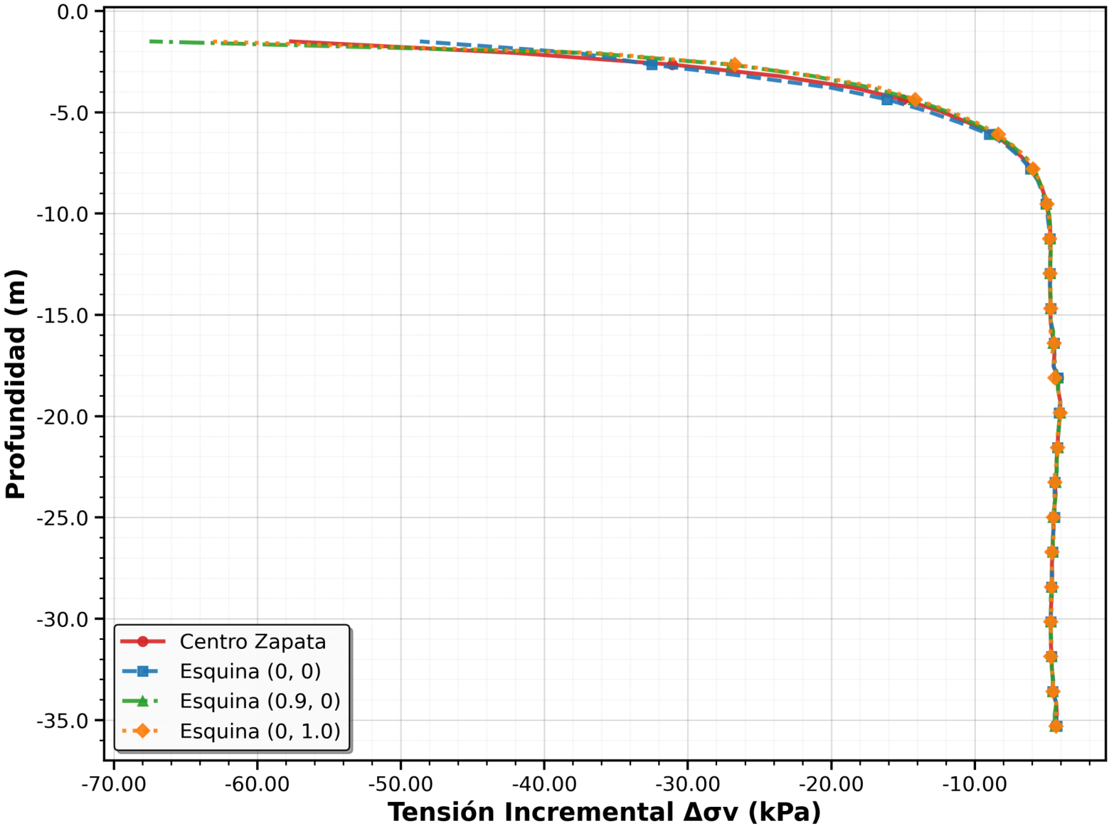
Perfiles Verticales de Tensiones Incrementales \Delta\sigma_v
