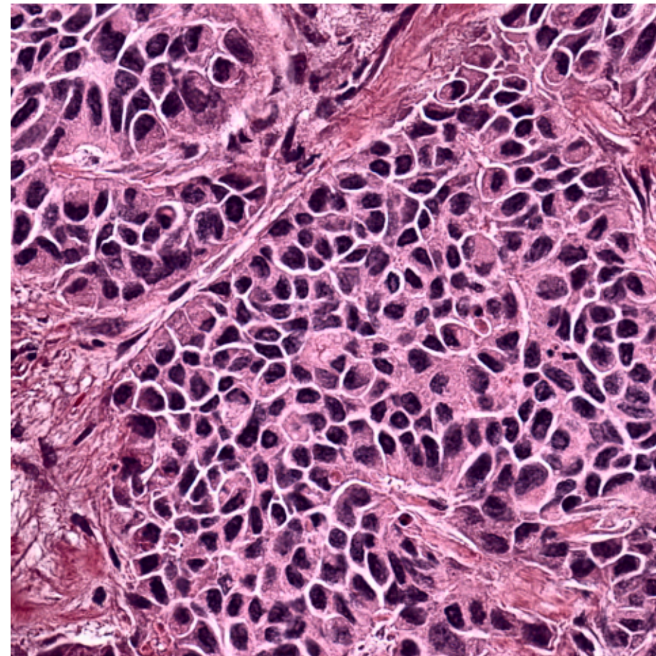
CLAHE
