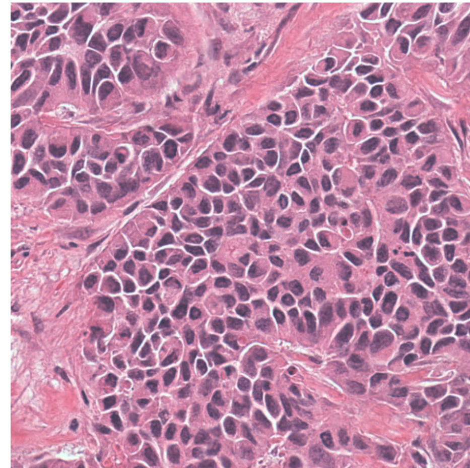
Reinhard
