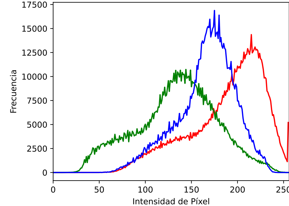
Reinhard
