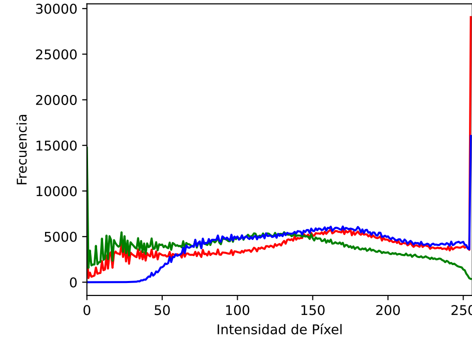
CLAHE
