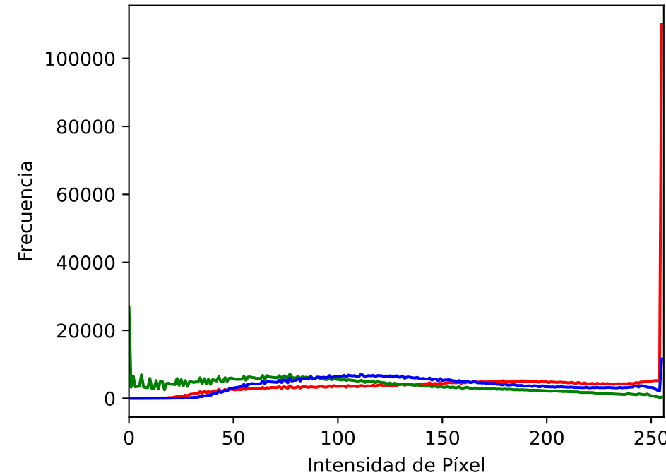
CLAHE
