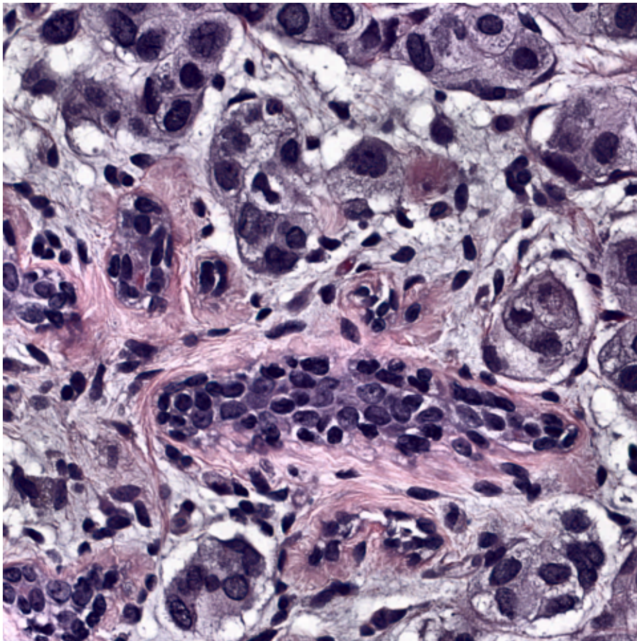
CLAHE
