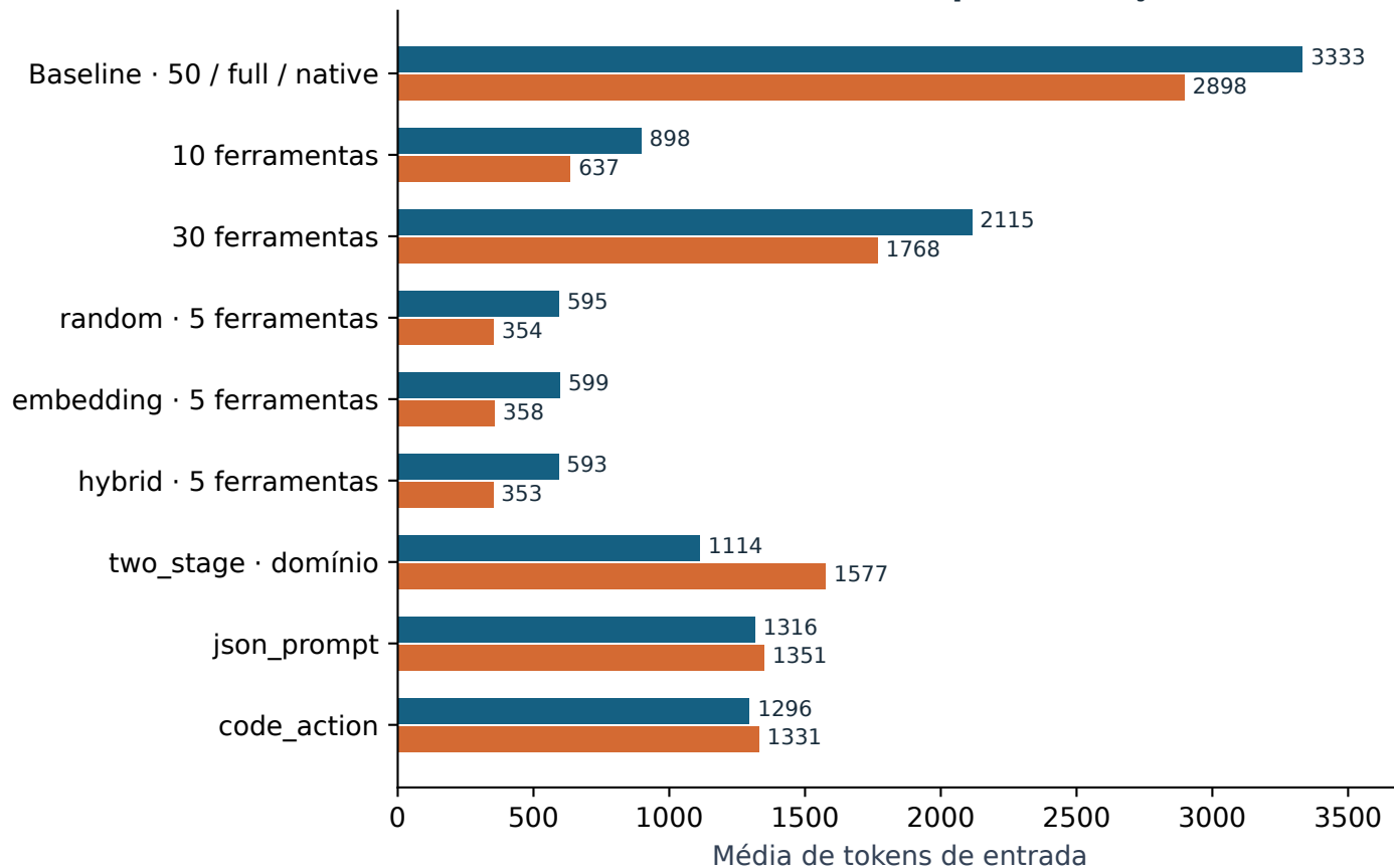
Tokens de entrada por execução
