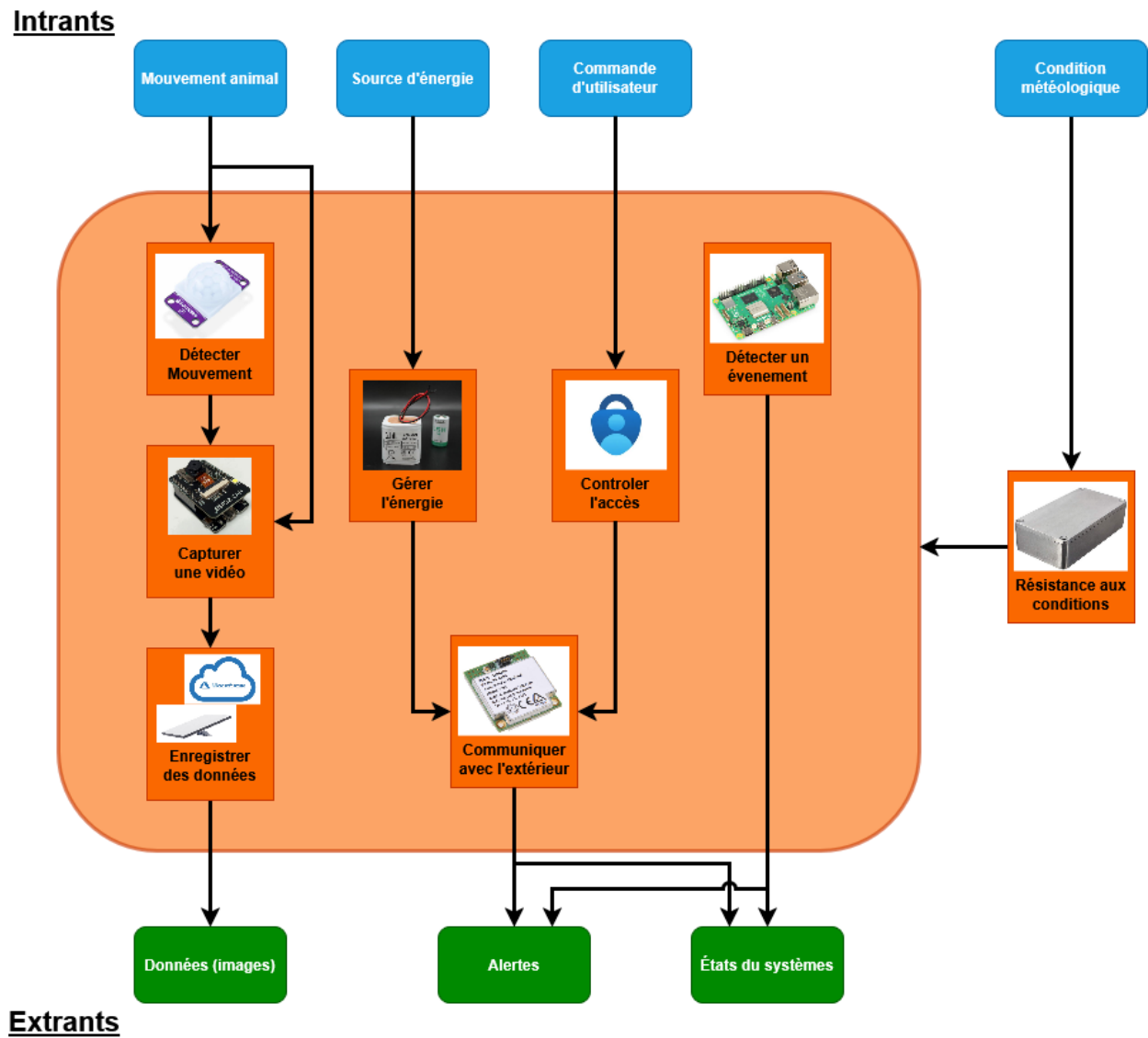
FIGURE 7.2 – Diagramme physique du projet NordFaune
