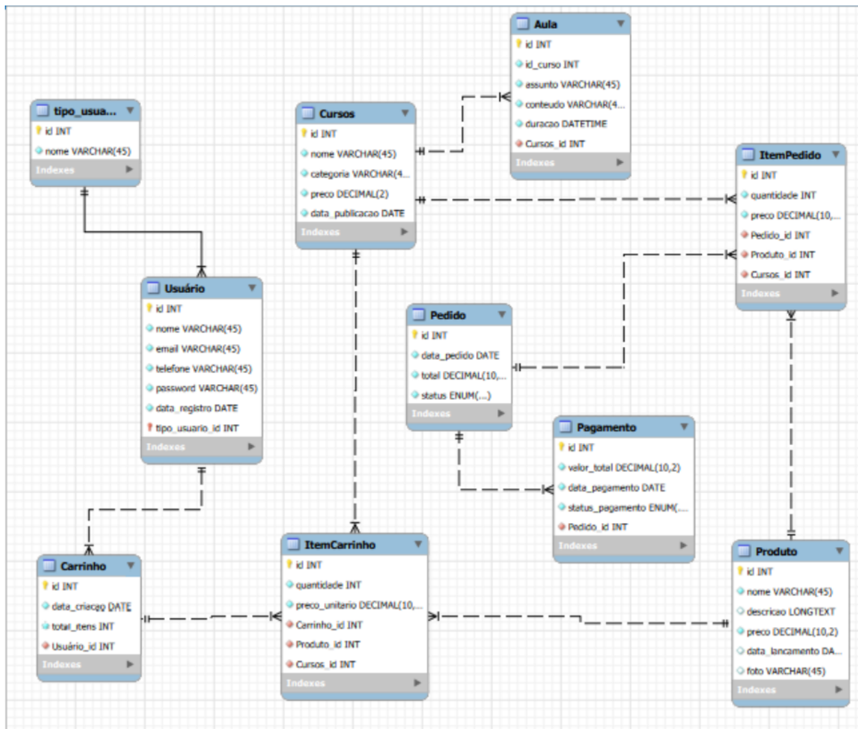
Figura2 – Modelo Entidade-Relacionamento
