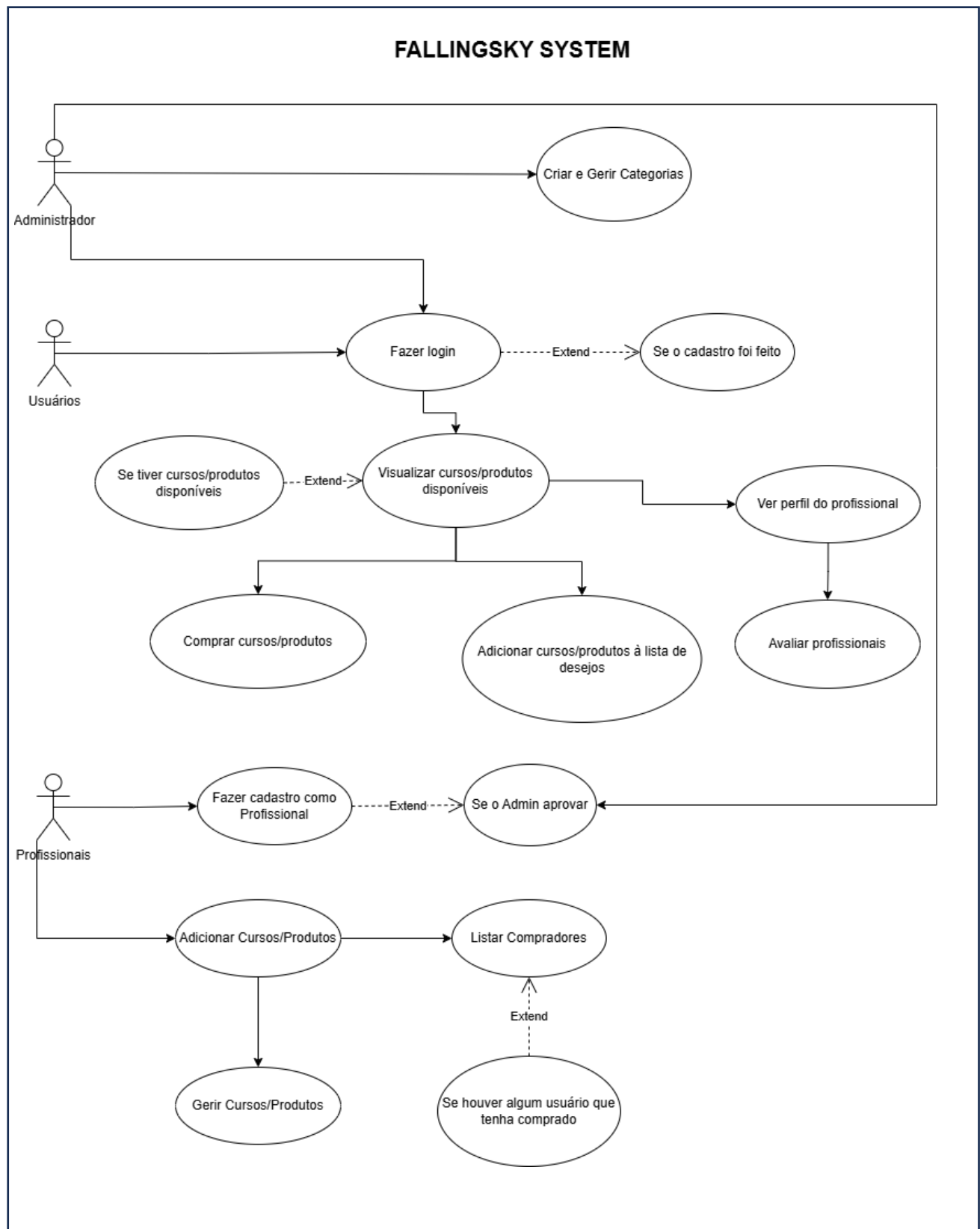
Figura1 – Diagrama de Use Case
