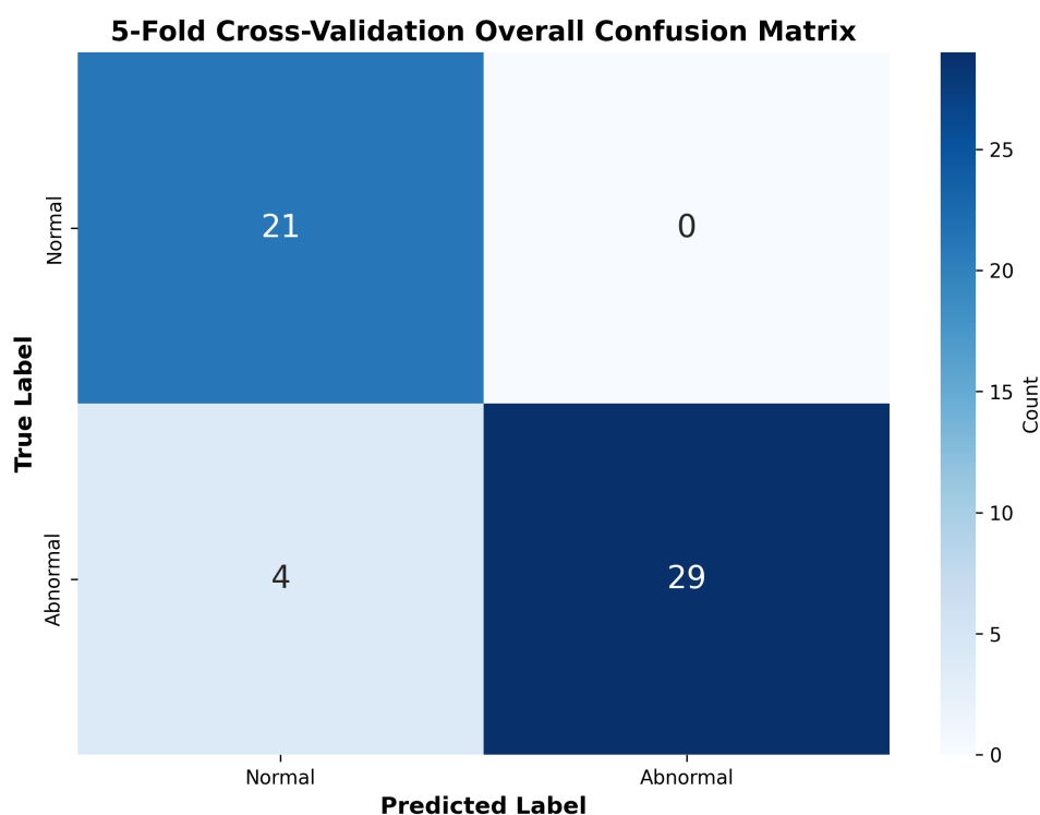
圖 4.1: RQ1 量化特徵二分類混淆矩陣圖
