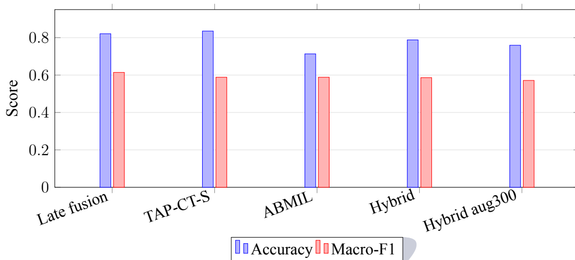
圖 4.4: 塌陷角三分類效能比較
