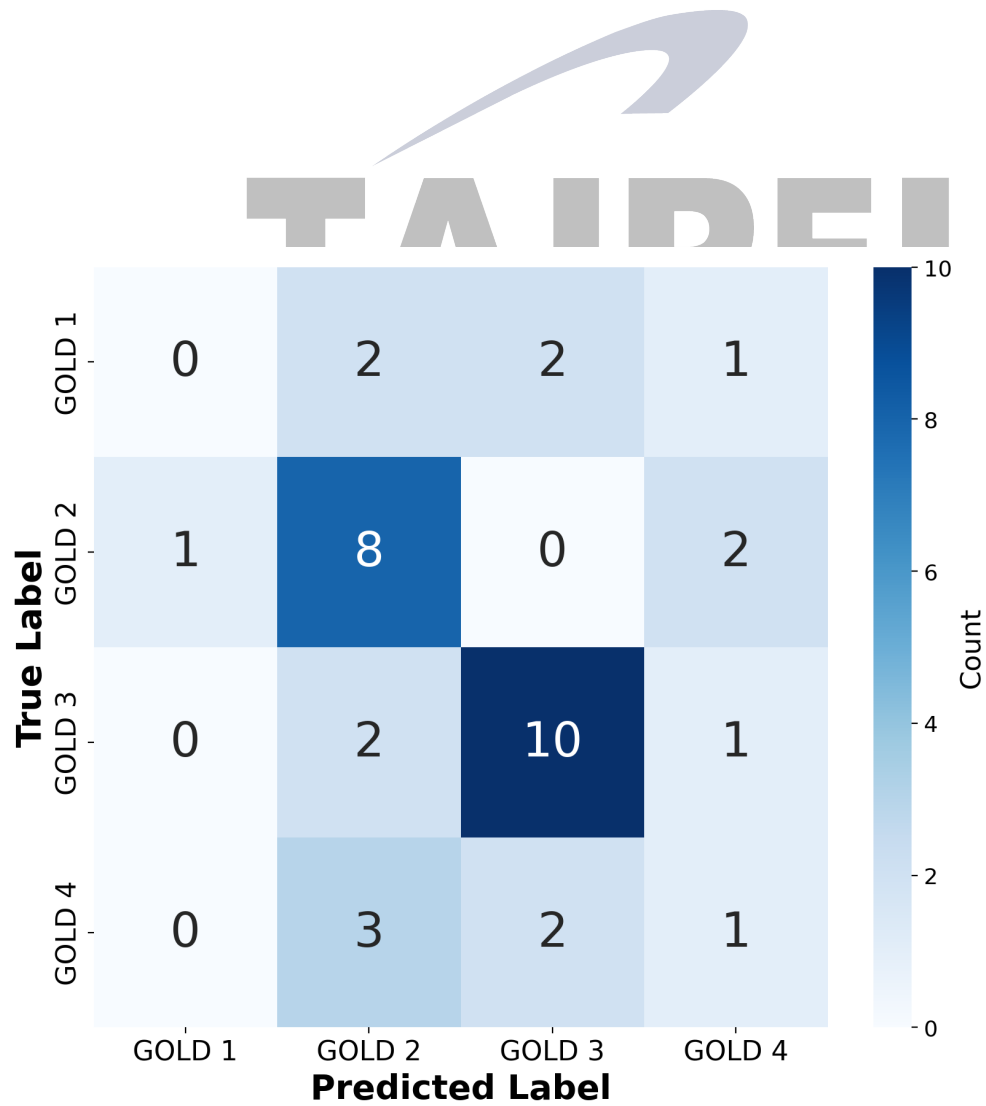
圖 4.4: RQ5 GOLD 四分級分類混淆矩陣
