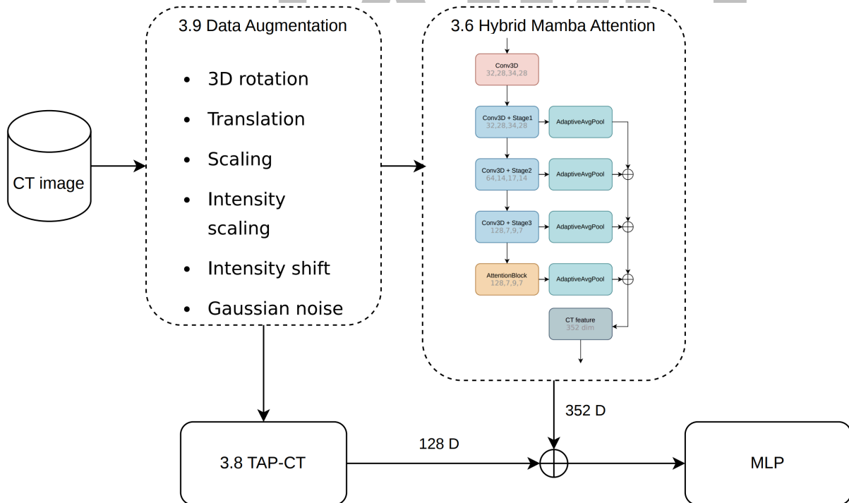
圖 3.2: 三維電腦斷層影像 TAP-CT 後期融合模型流程概覽（資料增強見 ?? 節、影像編碼器見 ?? 節、融合策略見 ?? 節）
