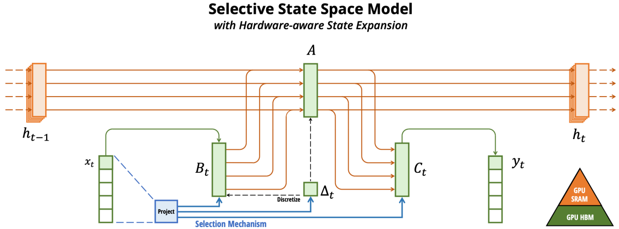
圖 2.2: 具選擇機制之狀態空間模型架構
