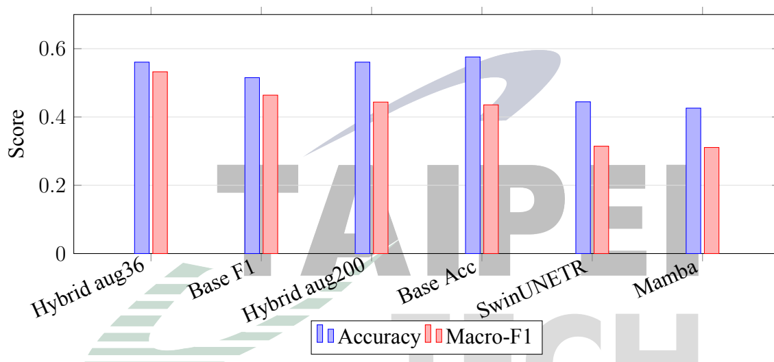
圖 4.5: 候選分級分類效能比較
