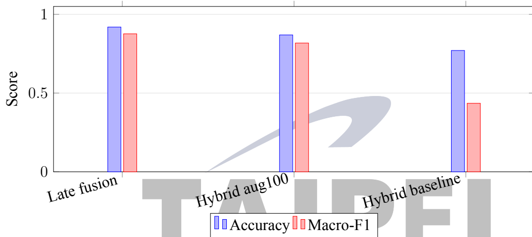
圖 4.3: 塌陷角二分類效能比較
