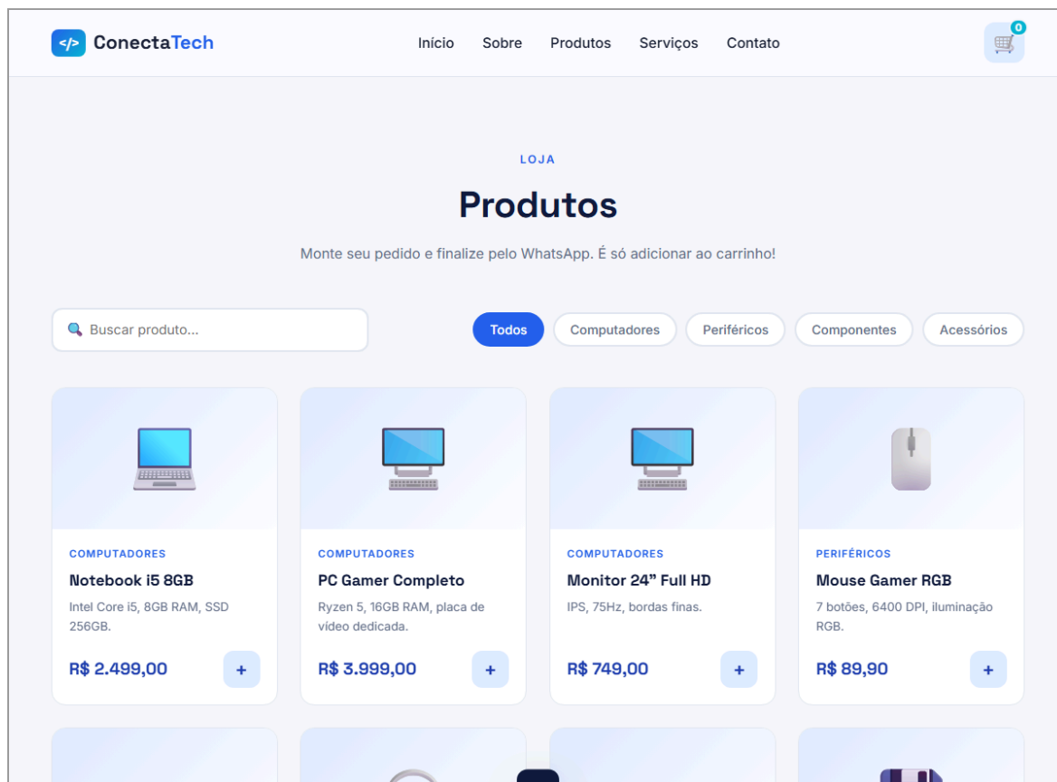
Figura 3: Catálogo de produtos com busca e filtro por categoria.
