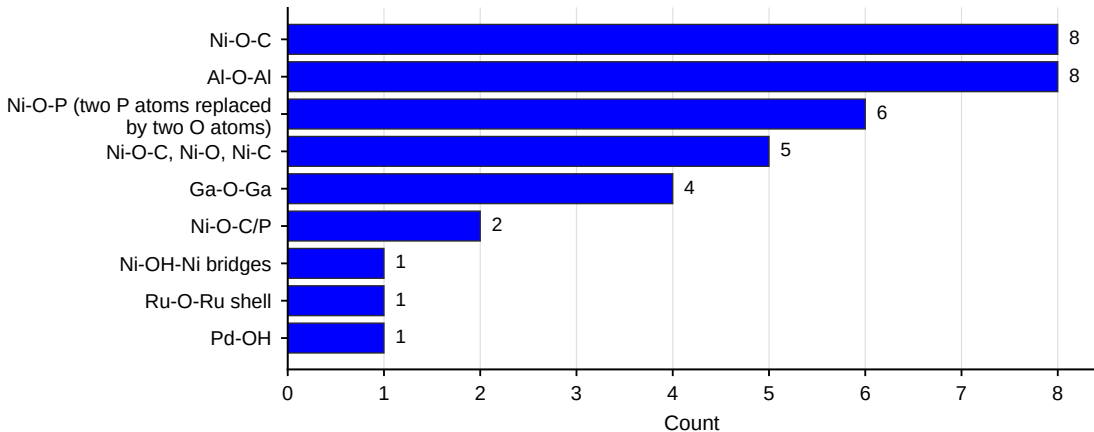
Top bridge/interface motifs
