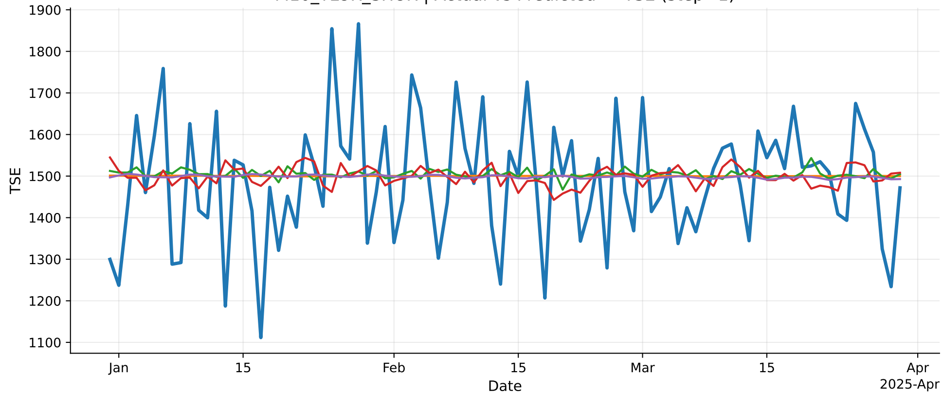
M10_YLUR_SHUR | Actual vs Predicted — TSE (step=1)
