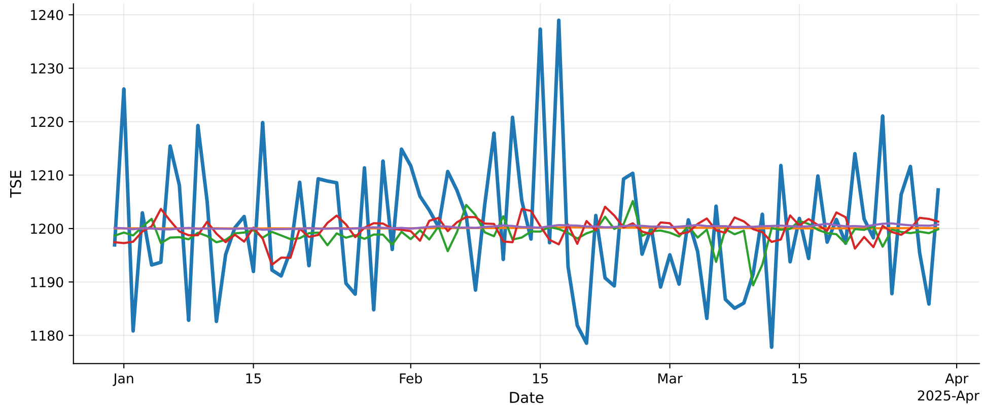
M8_YLUR_SLUR | Actual vs Predicted — TSE (step=1)
