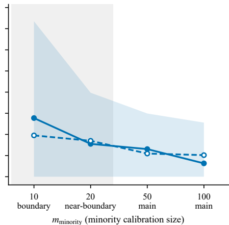
TabPFN
