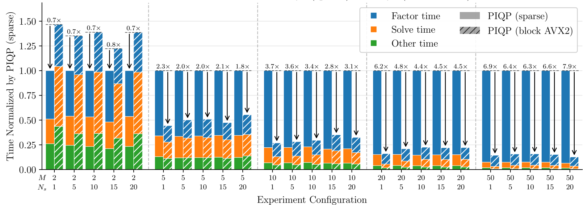
Solve Time Breakdown: PIQP (sparse) vs PIQP (block AVX2)
