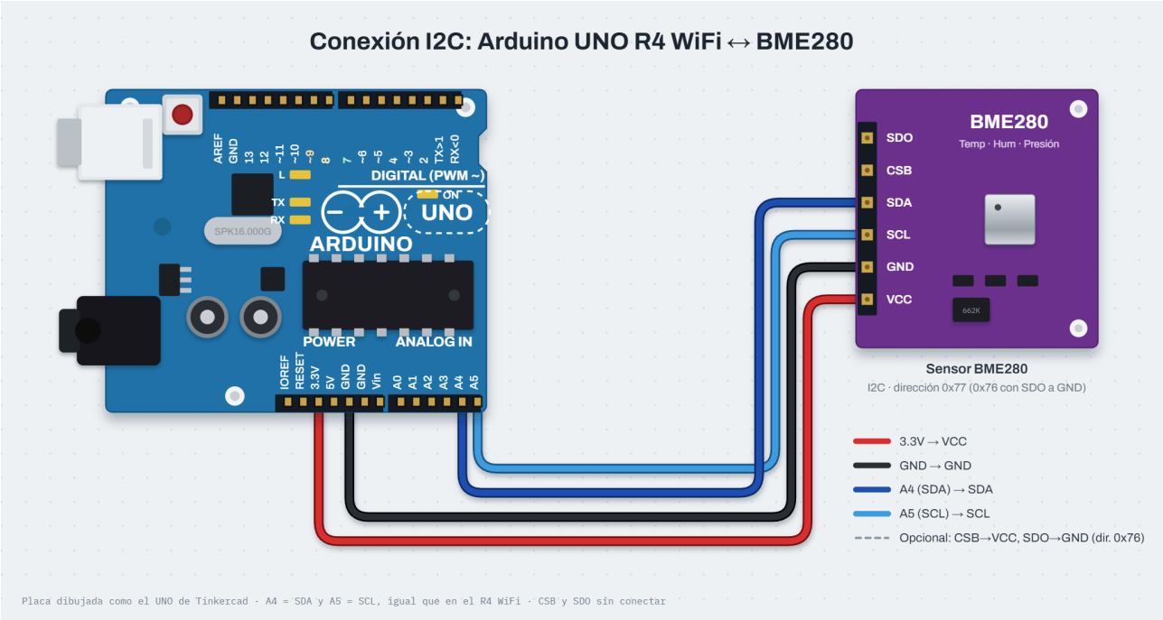
Diagrama de conexión: UNO R4 WiFi y sensor por I2C (A4 = SDA, A5 = SCL), alimentado a 3.3 V.
