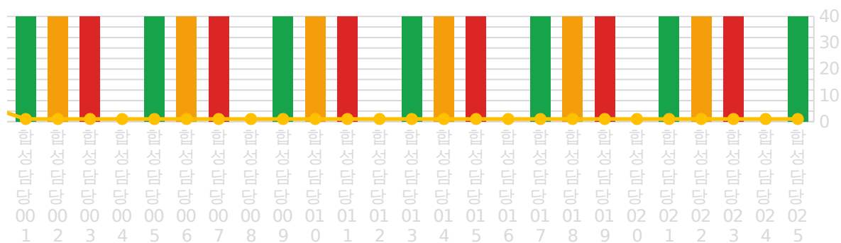
당자별 수용률 (1-40 / 100)
