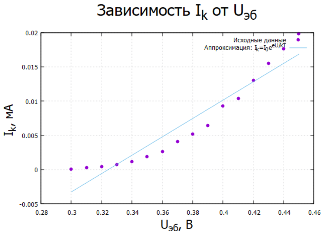
Рис. 2. Зависимость I_k от U
