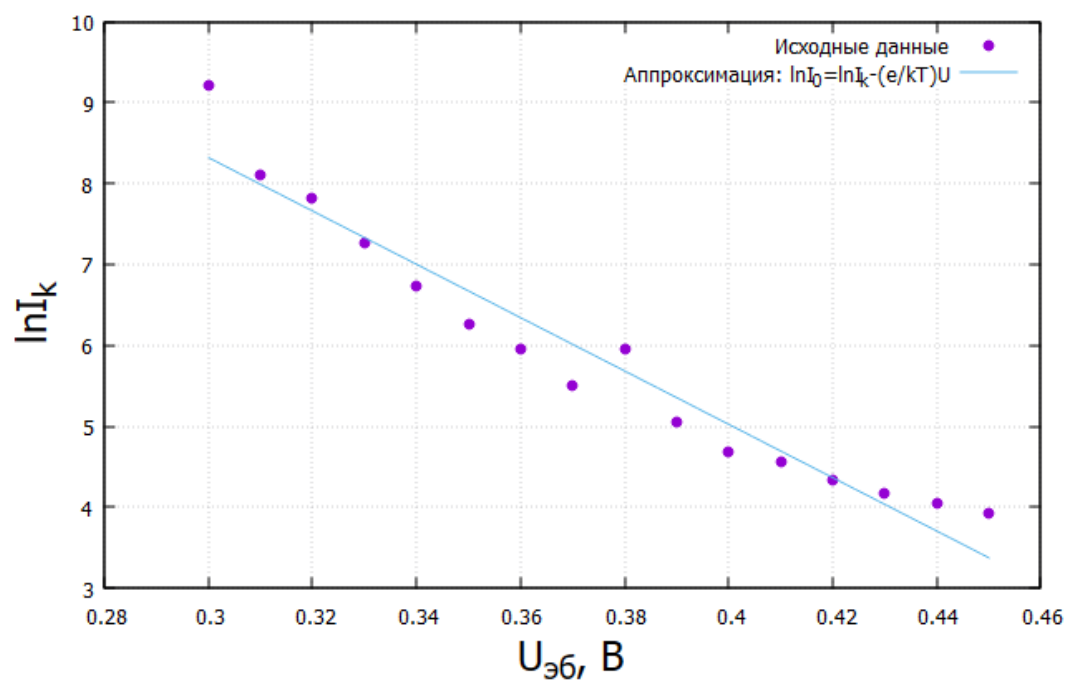
Рис. 3. Зависимость \ln I_k от U
