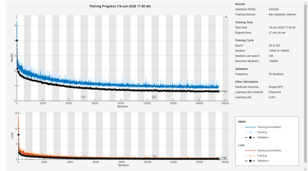
Entrenamiento del modelo de precio — parada en la época 29 de 200
