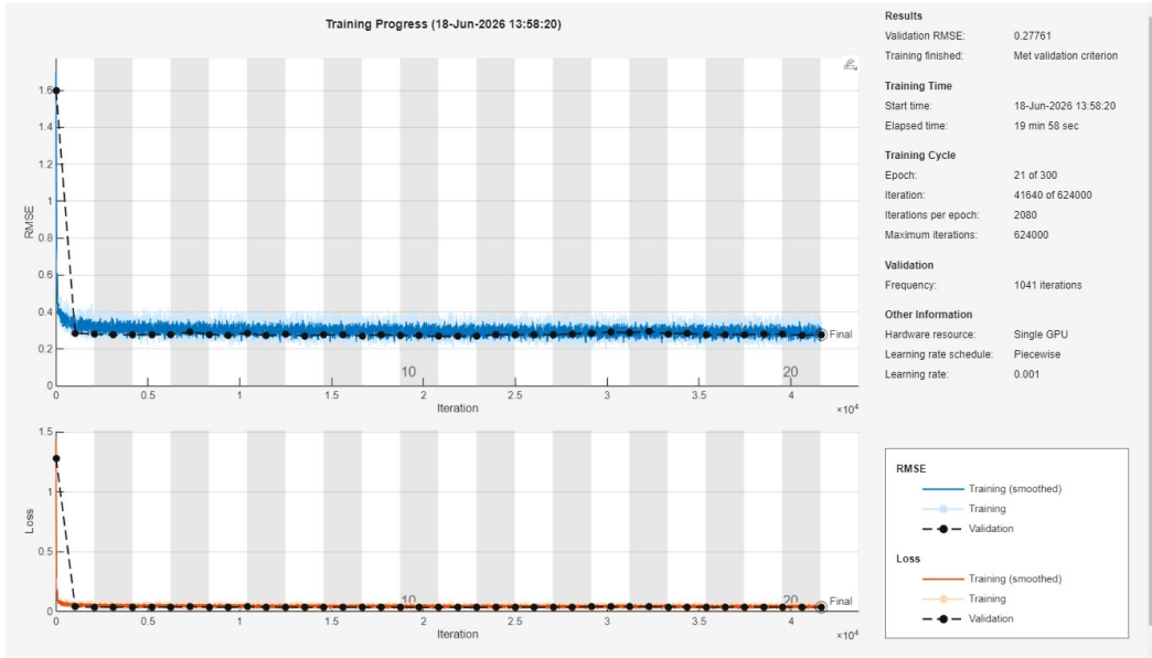
Entrenamiento del modelo solar — parada en la época 21 de 300
