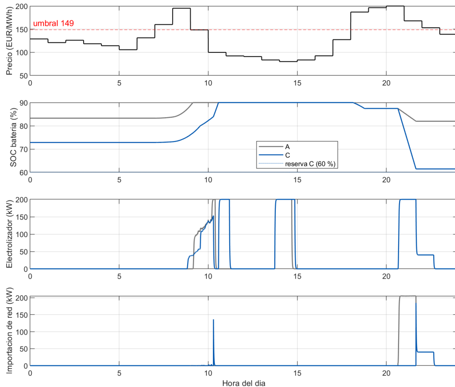
Figura 6.4: Un día del escenario nublado, hora a hora, para la misma semilla: precio, estado de carga de la batería, potencia del electrolizador e importación de red. En C la batería baja hasta la reserva del 60 % alimentando al electrolizador y la importación desaparece en esas horas; en A la batería se mantiene llena y el electrolizador consume red.
