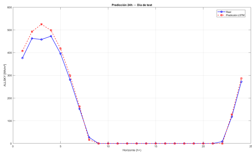
Figura 4.3: Predicción LSTM solar completa a 24 horas para un día de test. Cada punto corresponde a un horizonte h+1 , h+2 , ..., h+24 .
