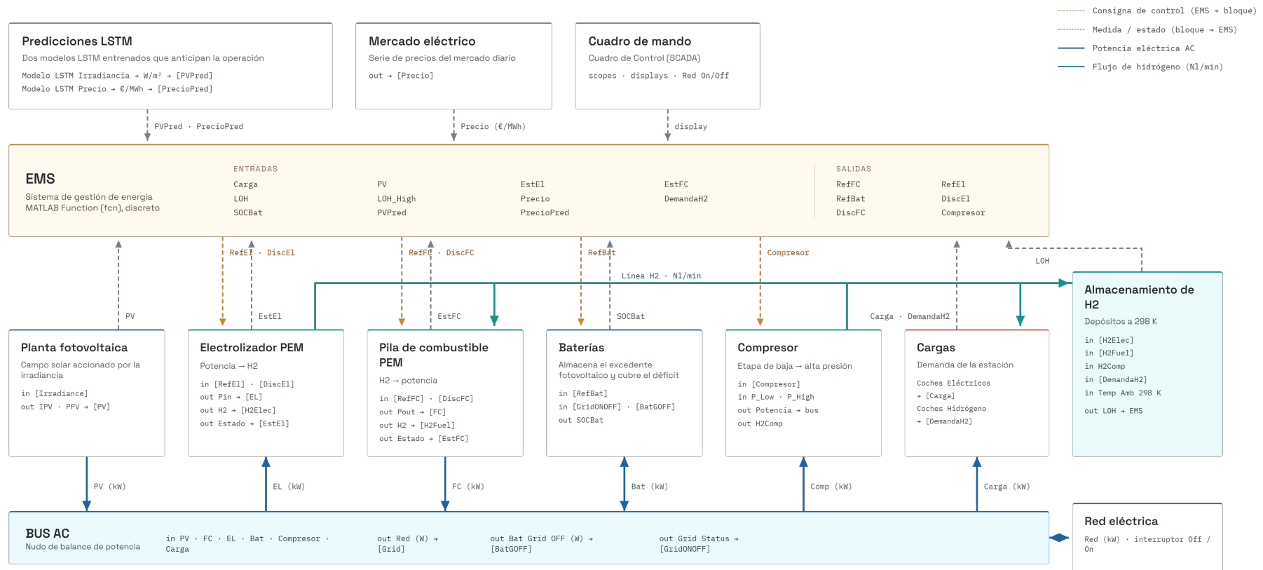
Figura 5.2: Arquitectura por módulos del modelo OASIS.slx. Los bloques se agrupan por la red que intercambian: consignas del EMS hacia los equipos (trazo discontinuo naranja), medidas de los equipos hacia el EMS (discontinuo gris), potencia eléctrica en el bus de alterna (azul) y flujo de hidrógeno (verde), con los nombres de las señales tal y como aparecen en Simulink. El EMS es un único bloque MATLAB Function con once entradas y seis salidas; las dos S-Functions de previsión le entregan PVPred y PrecioPred.
