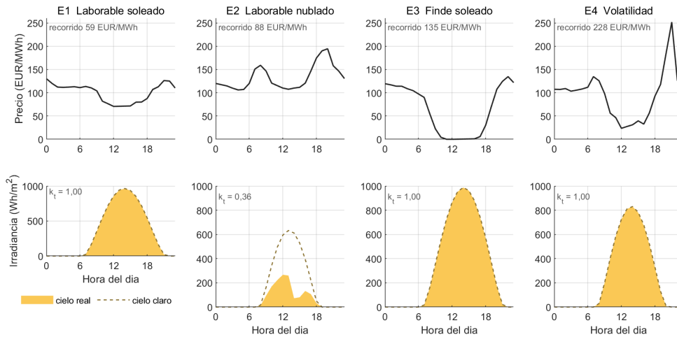
Figura 5.4: Los cuatro escenarios en su fecha: precio horario del mercado diario (arriba) e irradiancia horizontal real frente a la de cielo claro (abajo), con el índice de claridad k_t del día. Las cuatro columnas comparten escala, de modo que la comparación entre ellas es directa.
