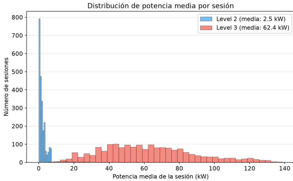
Figura 3.4: Distribución de potencia media por sesión: Level 2 vs Level 3.
