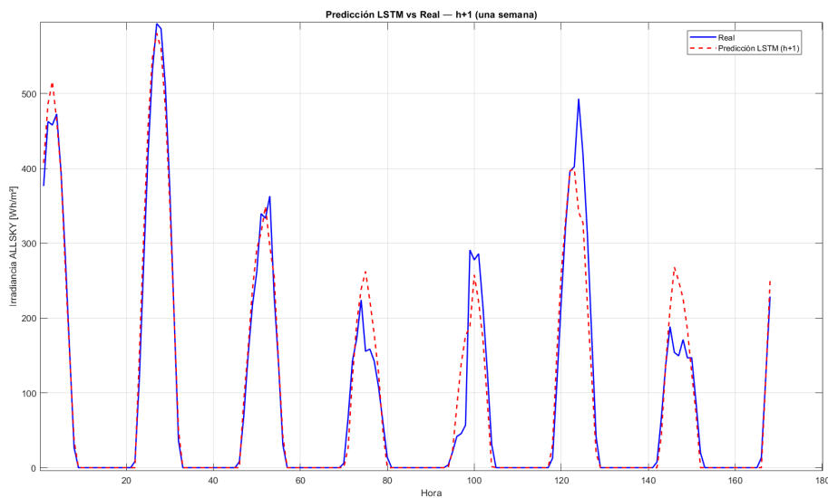
Figura 4.2: Predicción LSTM solar ( h+1 ) vs. irradiancia real ALLSKY durante una semana del conjunto de test (Sevilla, NASA POWER).
