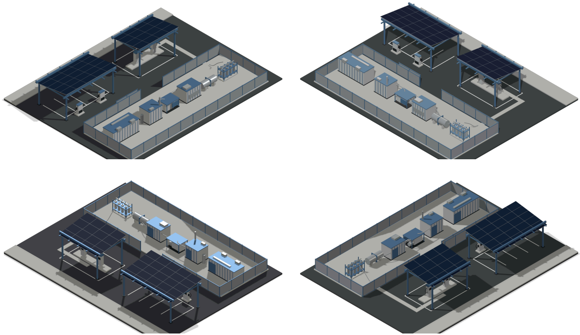
Figura 5.1: Vistas isométricas de la estación OASIS desde los cuatro cuadrantes (noroeste, noreste, suroeste y sureste). Las dos marquesinas fotovoltaicas cubren los dos cargadores de vehículo eléctrico de 50 kW y el surtidor de hidrógeno; el recinto vallado agrupa los contenedores de batería, electroliizador, compresor y pila de combustible, el tanque tampón de baja presión y el bastidor de botellas de alta presión.
