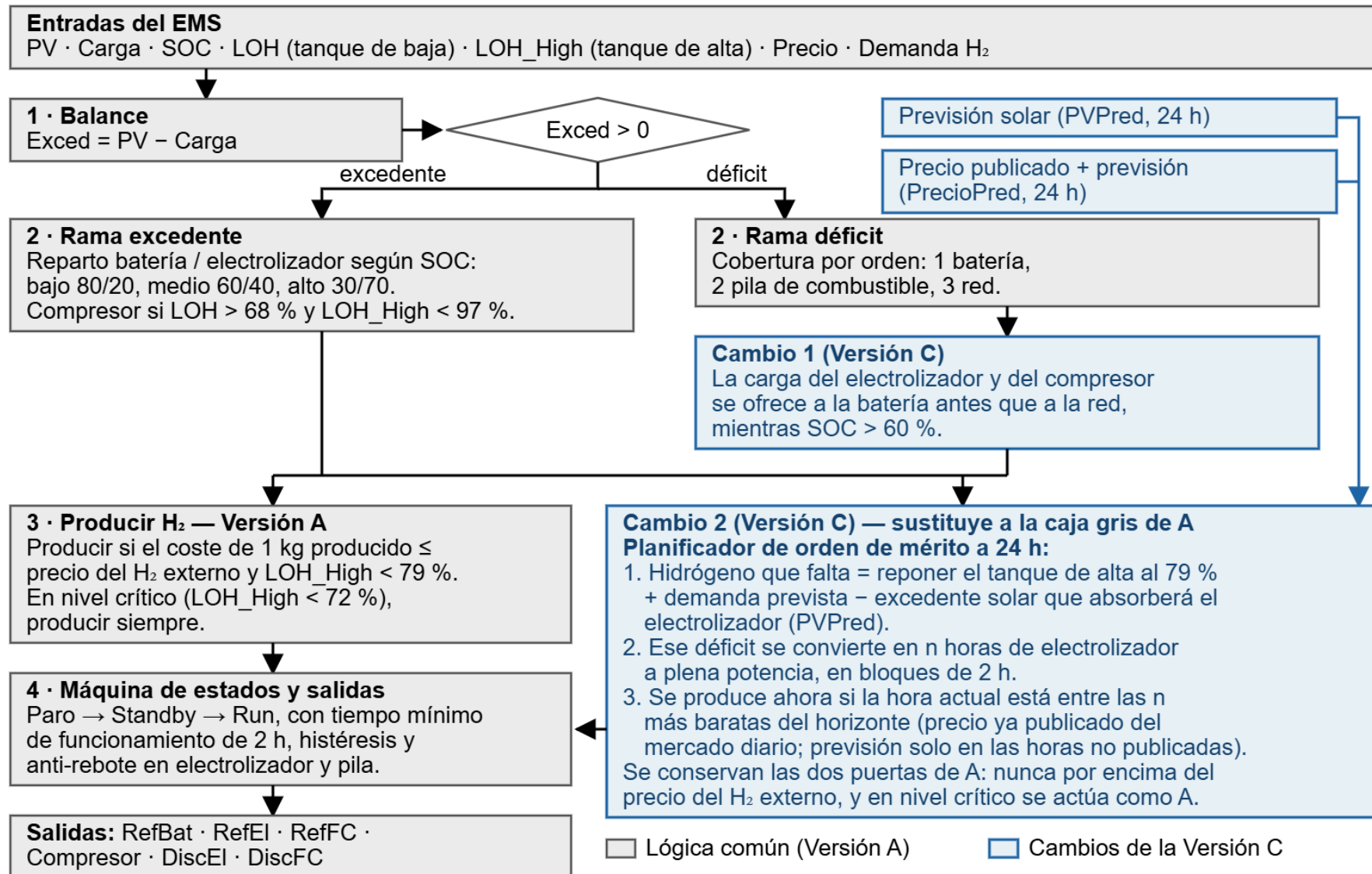
Figura 5.3: Lógica de decisión del EMS. En gris, la lógica común heredada de la Versión A: balance, reparto por estado de carga en la rama de excedente, cobertura del déficit por orden de mérito, decisión económica de producir hidrógeno y máquina de estados. En azul, los dos únicos cambios de la Versión C: la carga del electrolizador y del compresor se ofrece a la batería antes que a la red, y la decisión de producir pasa a ser un planificador de orden de mérito a 24 h que consume el precio publicado del mercado diario, la previsión de precio en las horas no publicadas y la previsión solar. La variante predictiva inyectaba las previsiones en los bloques 2 y 3 de A y no se representa.
