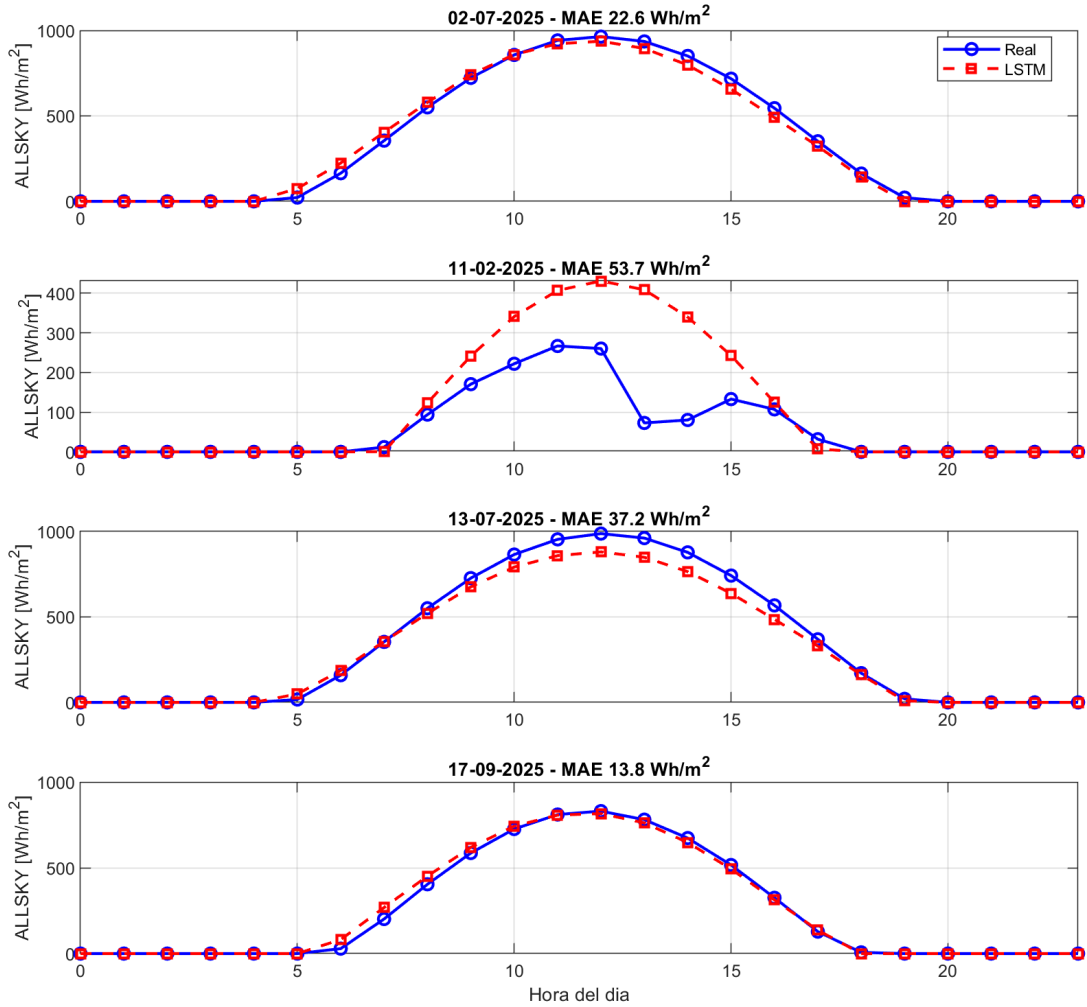
Figura 4.4: Predicción de irradiancia frente al valor real de NASA POWER en los cuatro días de la campaña de simulación.
