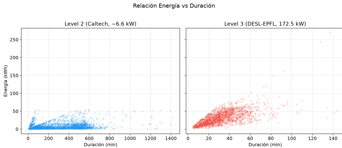
Figura 3.5: Relación energía vs duración: Level 2 (izq) vs Level 3 (der).
