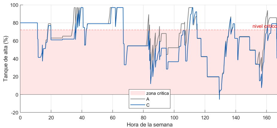
Figura 6.5: Nivel del tanque de alta a lo largo de la semana nublada, misma semilla, con la zona crítica sombreada. C pasa más tiempo en la zona crítica que A.
