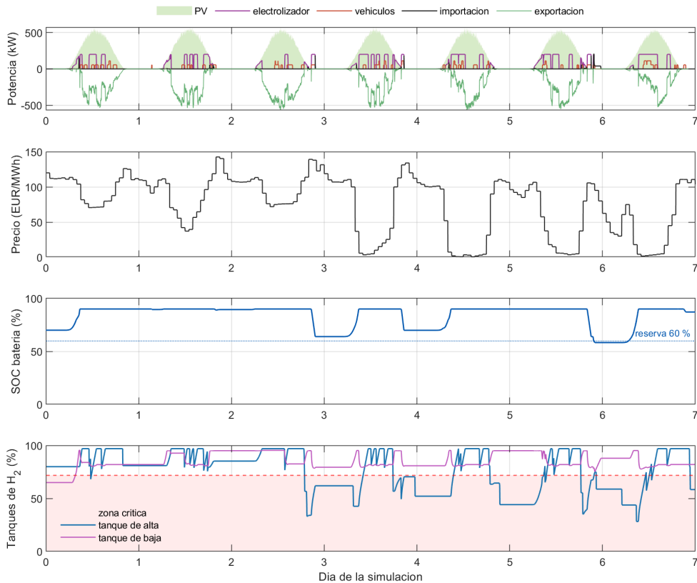
Figura 6.1: Una semana completa del escenario laborable soleado con la Versión C, semilla 1. De arriba abajo: potencias en el bus de alterna (fotovoltaica, electrolizador, carga de vehículos, importación y exportación de red), precio horario del mercado diario, estado de carga de la batería con su reserva del 60 % y nivel de los dos tanques de hidrógeno con la zona crítica sombreada.
