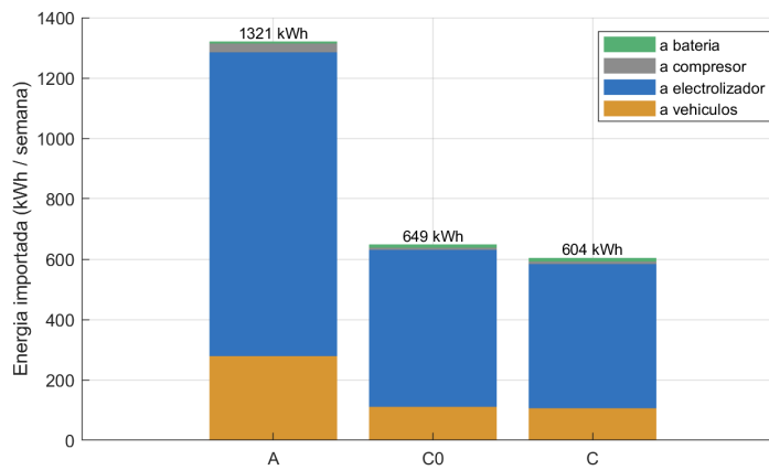
Figura 6.2: Destino de la energía importada de la red, media semanal, para la Versión A y para las dos etapas de la Versión C. En A tres cuartas partes van al electrolizador; en C ese bloque se reduce a la mitad porque lo alimenta la batería.
