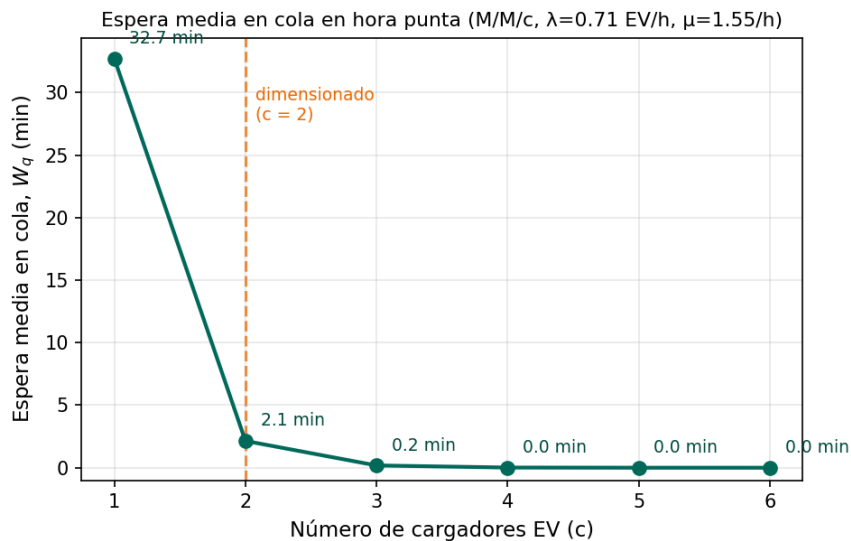
Figura 3.7: Espera media en cola W_q (Erlang C) frente al número de cargadores, para \lambda = 0.71 \text{ EV/h} y \mu = 1.55 servicios/h. El salto entre c = 1 y c = 2 (de \approx 33 \text{ min} a \approx 2 \text{ min} ) sustenta la elección de 2 cargadores; a partir de c = 3 la mejora es marginal.
