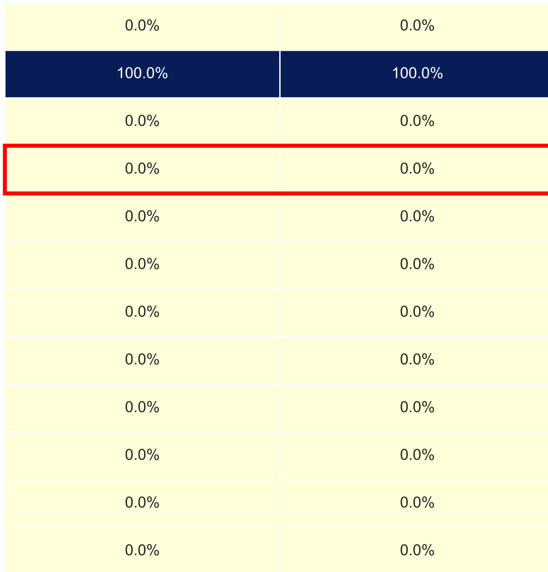
Posterior Weight Evolution: OLS BMA (BIC-W) ( p_0 = 4 )
