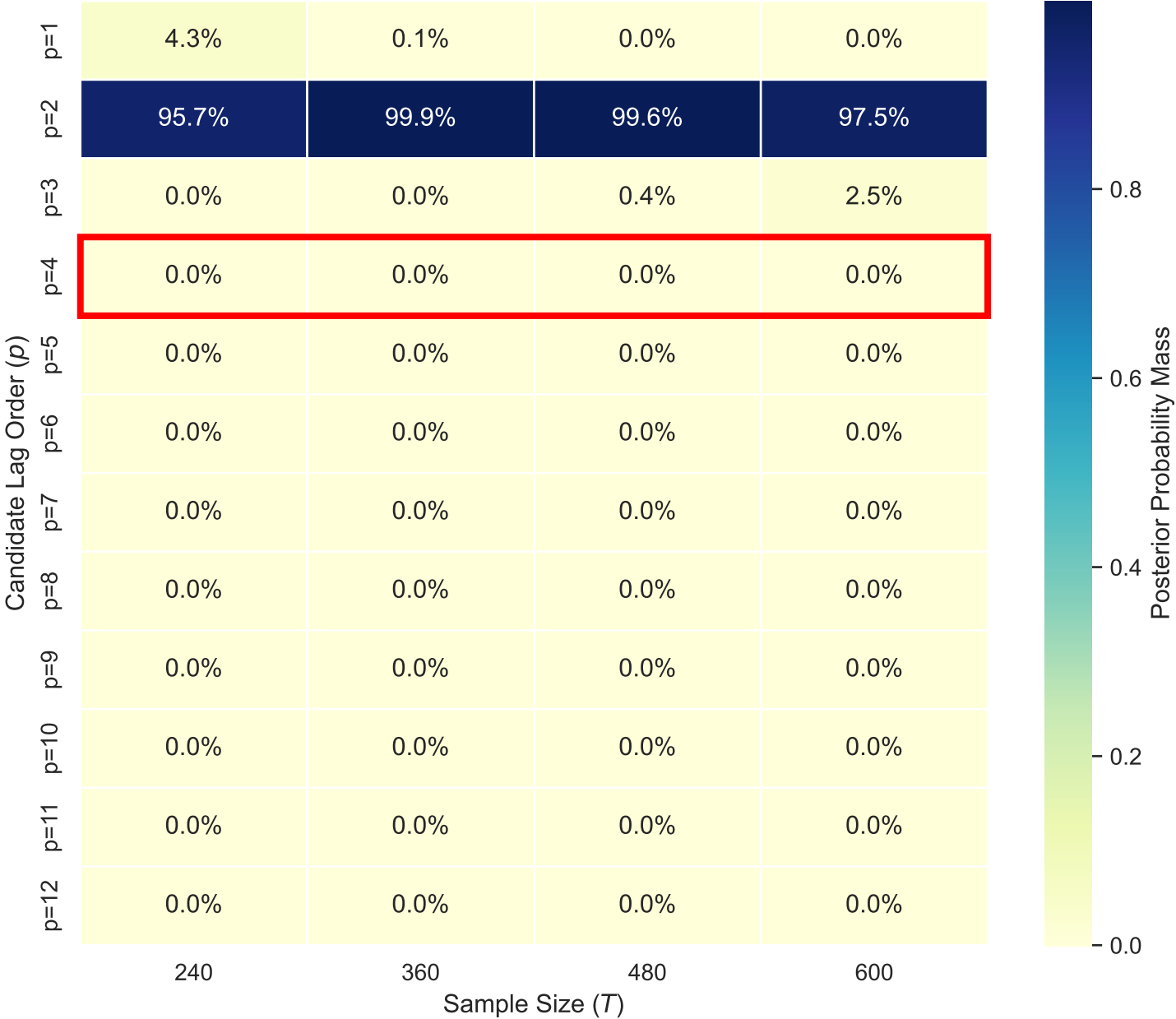
Posterior Weight Evolution: OLS BMA (BIC-W) ( p_0 = 4 )
