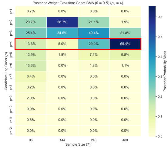
(d) Geom BMA ( \theta = 0.5 )
