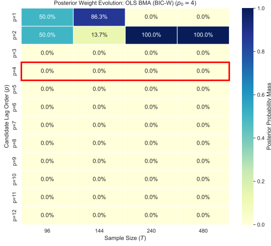
(a) OLS BMA (BIC-W)
