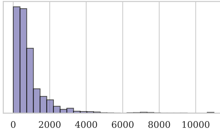
transport_co2 (Skew: 4.20)
