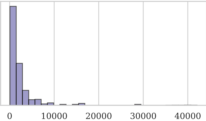
pop_density (Skew: 5.51)
