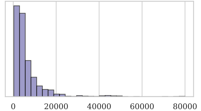
total_co2 (Skew: 4.14)
