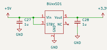
Régulateur 3.3V
