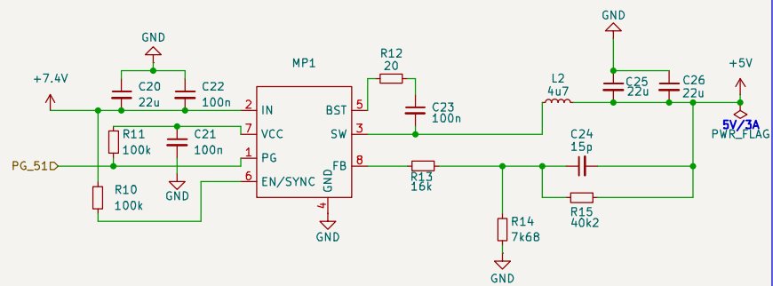
Régulateur 5V/3A
