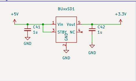
Régulateur 3.3V
