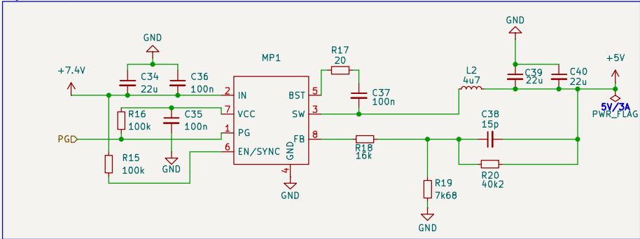
Régulateur 5V/3A
