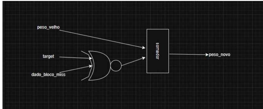
Figura 5: Lógica combinacional da função de treino: atualização de pesos via porta XNOR e somador.
