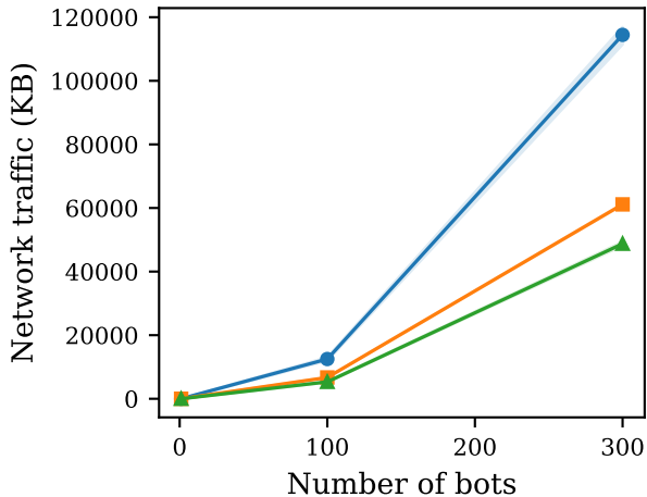
Local (0 ms)
