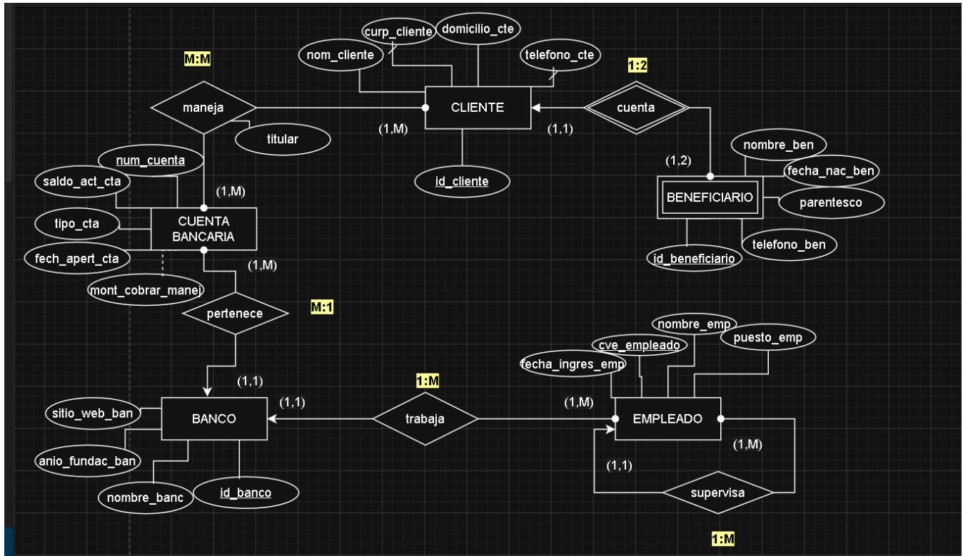
Figura 1: Modelo entidad relacion ejercicio 4_2
