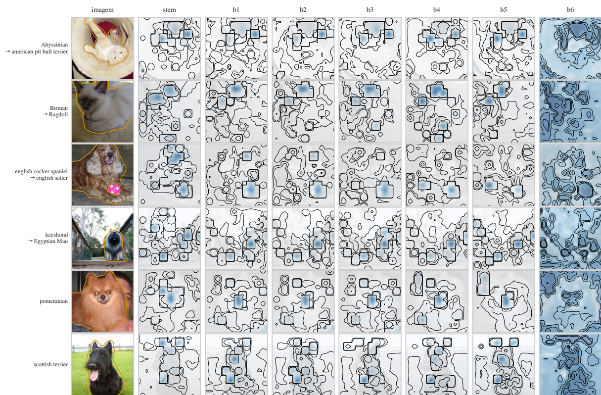
Figura 13: Campo de energia da Gram conjunta do transformador sobre as mesmas imagens da Figura 8. O aspecto quadriculado vem da grade de tokens ( 16 \times 16 ), ampliada para a imagem. No último bloco, a cabeça é um pooling médio seguido de uma camada linear, de modo que o gradiente é o mesmo em todas as posições e o campo deixa de distinguir regiões.
