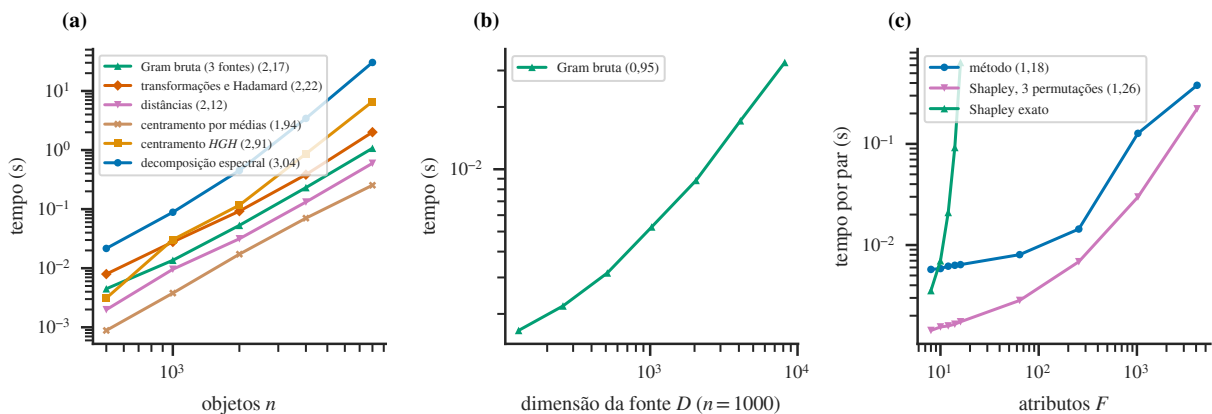
Figura 16: Tempo das etapas do método em função do tamanho do problema, em escala logarítmica nos dois eixos. Entre parênteses está a inclinação ajustada nos três maiores tamanhos, que estima o expoente do custo. (a) Etapas da construção e das leituras em função do número de objetos n , com três fontes de dimensão 256. (b) Matriz de Gram bruta em função da dimensão D da fonte, com n = 1000 . (c) Leitura de diferenças entre pares em função do número de atributos F , comparada ao valor de Shapley exato com j de referência e à sua estimativa por três permutações.
