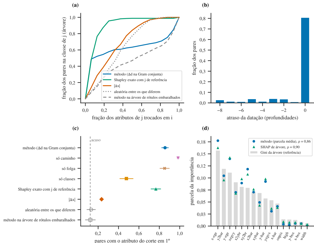
Figura 15: O método aplicado a uma árvore de decisão na letter . (a) Teste de trocas na própria árvore. (b) Diferença entre a profundidade em que o atributo de separação passa a ser o primeiro do método e a profundidade em que os caminhos de i e j se separam. (c) Fração dos pares em que o atributo de separação é o primeiro de cada ranking. (d) Importância global normalizada, na ordem da importância de Gini da árvore.
