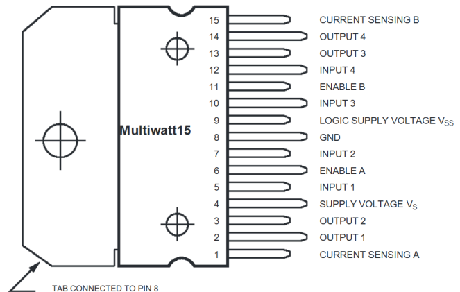
Fig. 3 Pinout L298N
