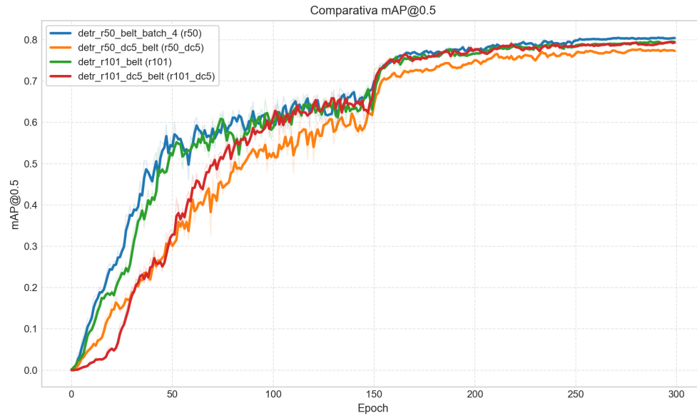
Figura 4.3.20: Precisión Media Promedio (mAP) vs época con umbral IoU 0,5 para todas las variantes del modelo DETR.
