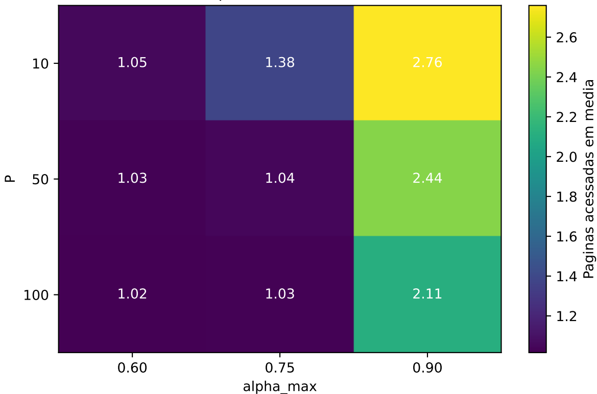
Heatmap: buscas com sucesso
