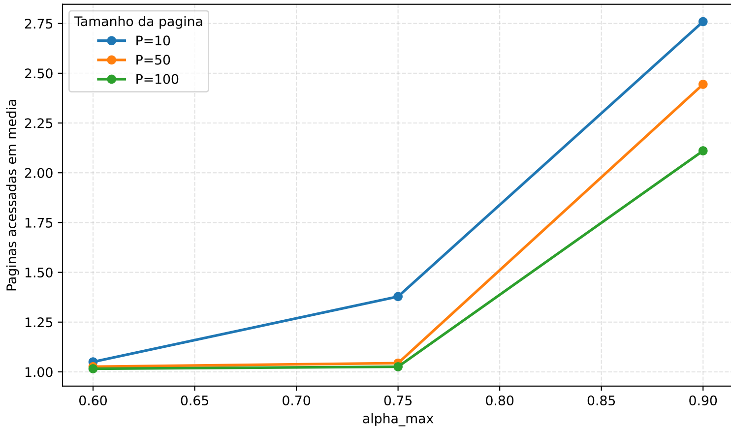
Custo medio de buscas com sucesso
