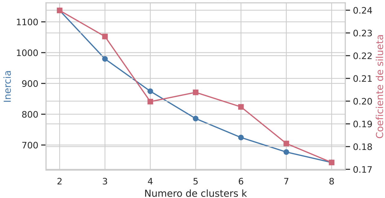
Metodo del codo y silueta para K-Means
