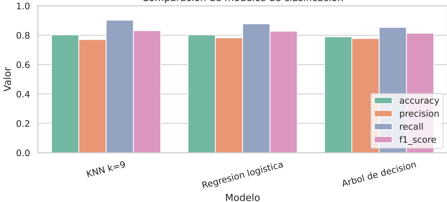
Comparacion de modelos de clasificacion
