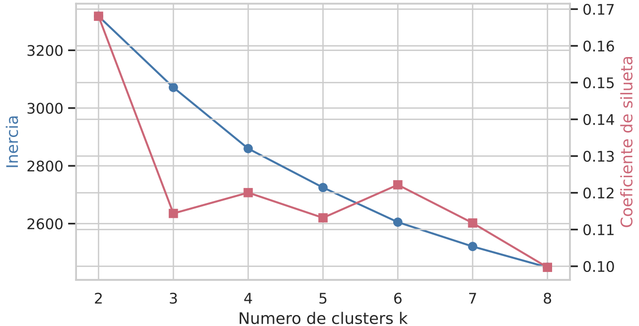
Metodo del codo y silueta para K-Means
