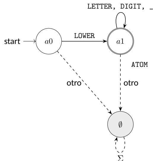
Figura 1: Autómata para átomos no entrecomillados.
