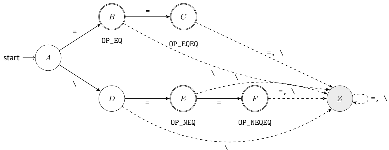
Figura 9: AFD mínimo etiquetado, con estado sumidero.
